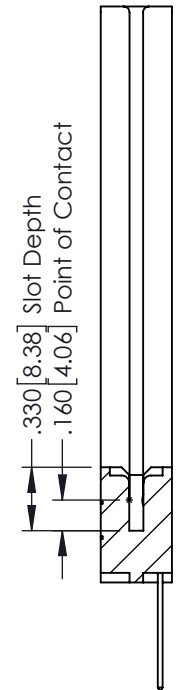
SECTION A-A
