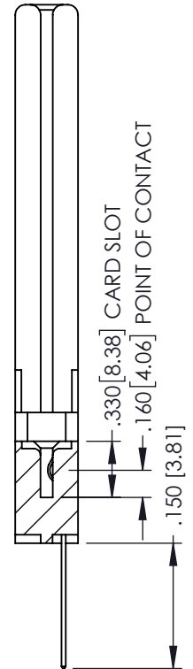
SECTION A-A
