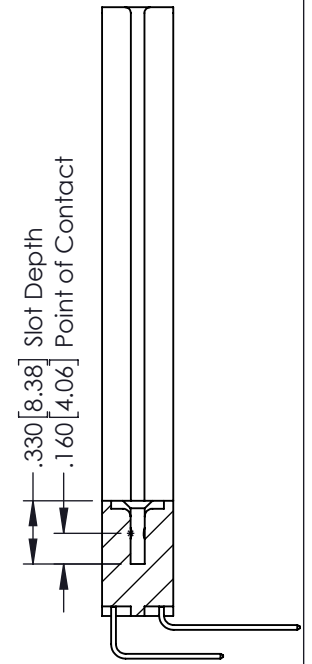
SECTION A-A
