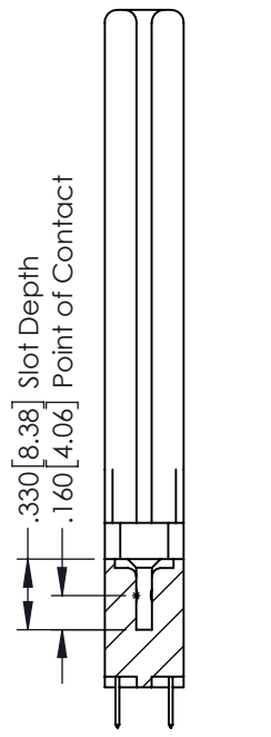
SECTION A-A
