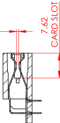
SECTION A-A SCALE 3 : 2
