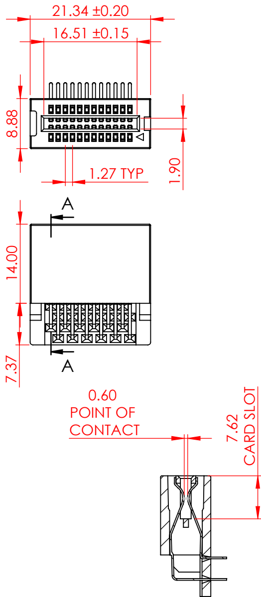
SECTION A-A SCALE 3 : 2
