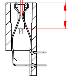
SECTION A-A SCALE 3 : 2
