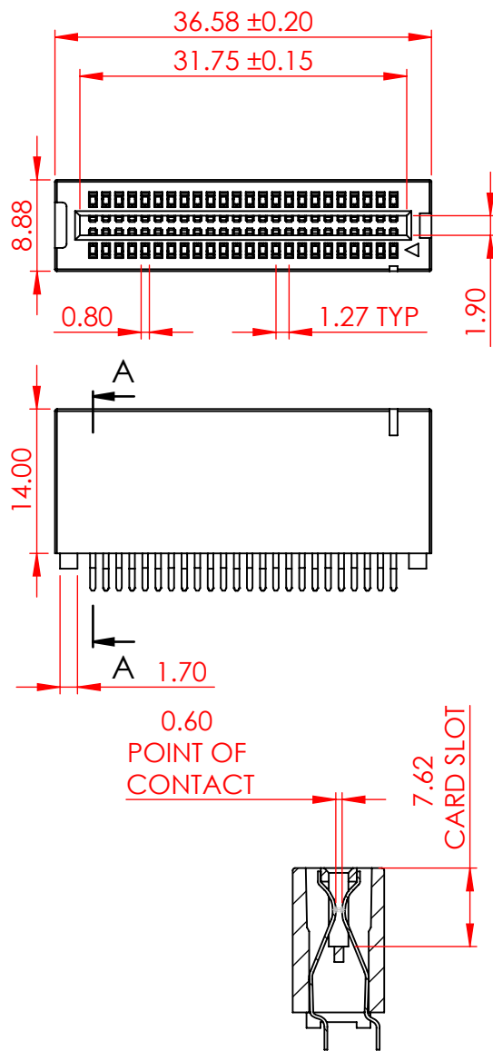
SECTION A-A SCALE 3 : 2
