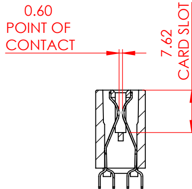
SECTION A-A SCALE 3 : 2
